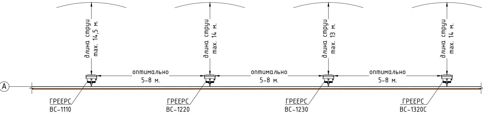
Максимальная длина потока воздуха и рекомендуемые расстояния между тепловентиляторами ГРЕЕРС ВС-1110/1220/1230/1320С
