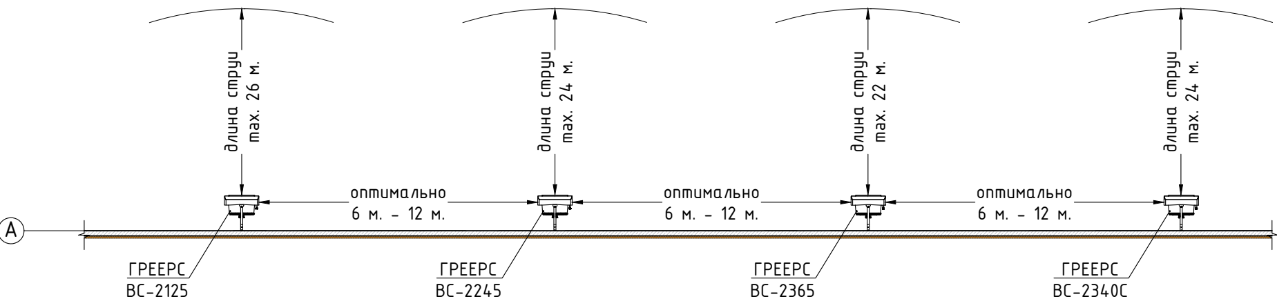
Максимальная длина потока воздуха и рекомендуемые расстояния между тепловентиляторами ГРЕЕРС ВС-2125/2245/2365/2340С
